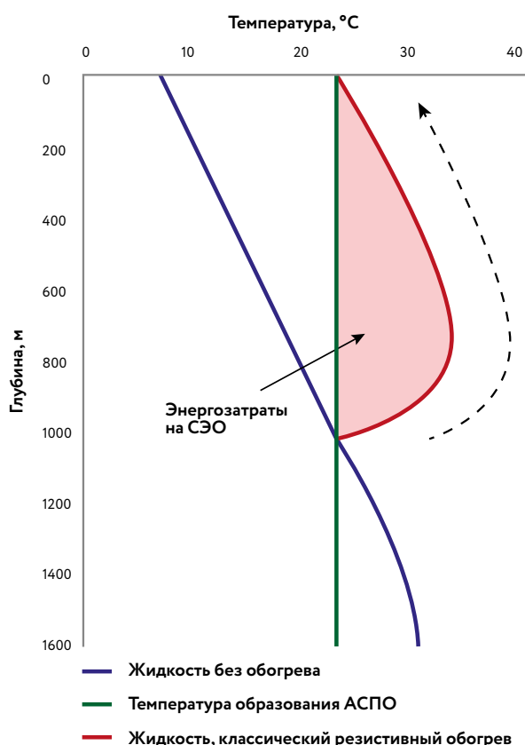
Распределение температуры флюида по глубине скважины при обогреве резистивным кабелем.
