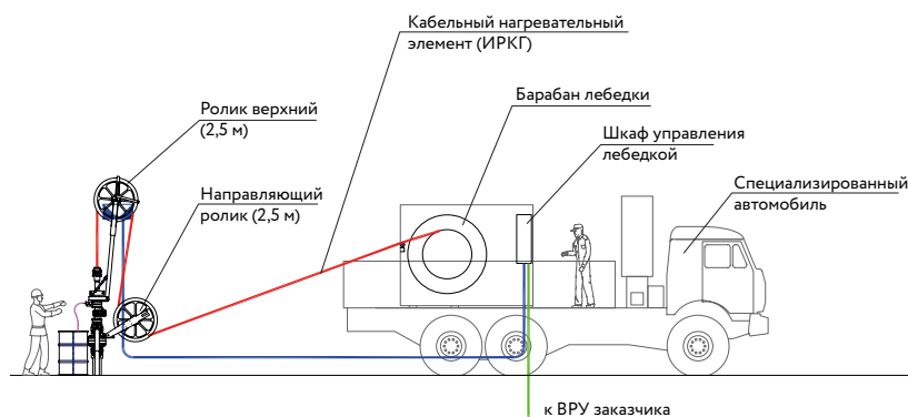
Схема расстановки спускоподъемного оборудования комплекса Stream Tracer
