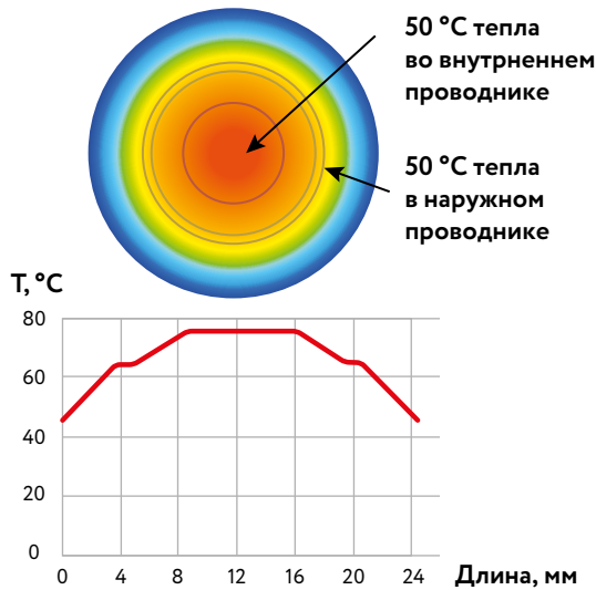
Тепловыделение нагревателя комплекса Stream Tracer
