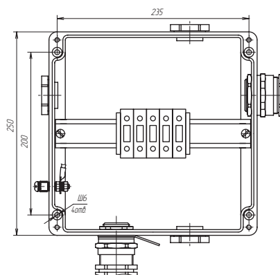
Коробка РТВ 1007
