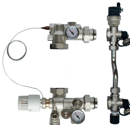
Смесительный узел Stahlmann Simplex
