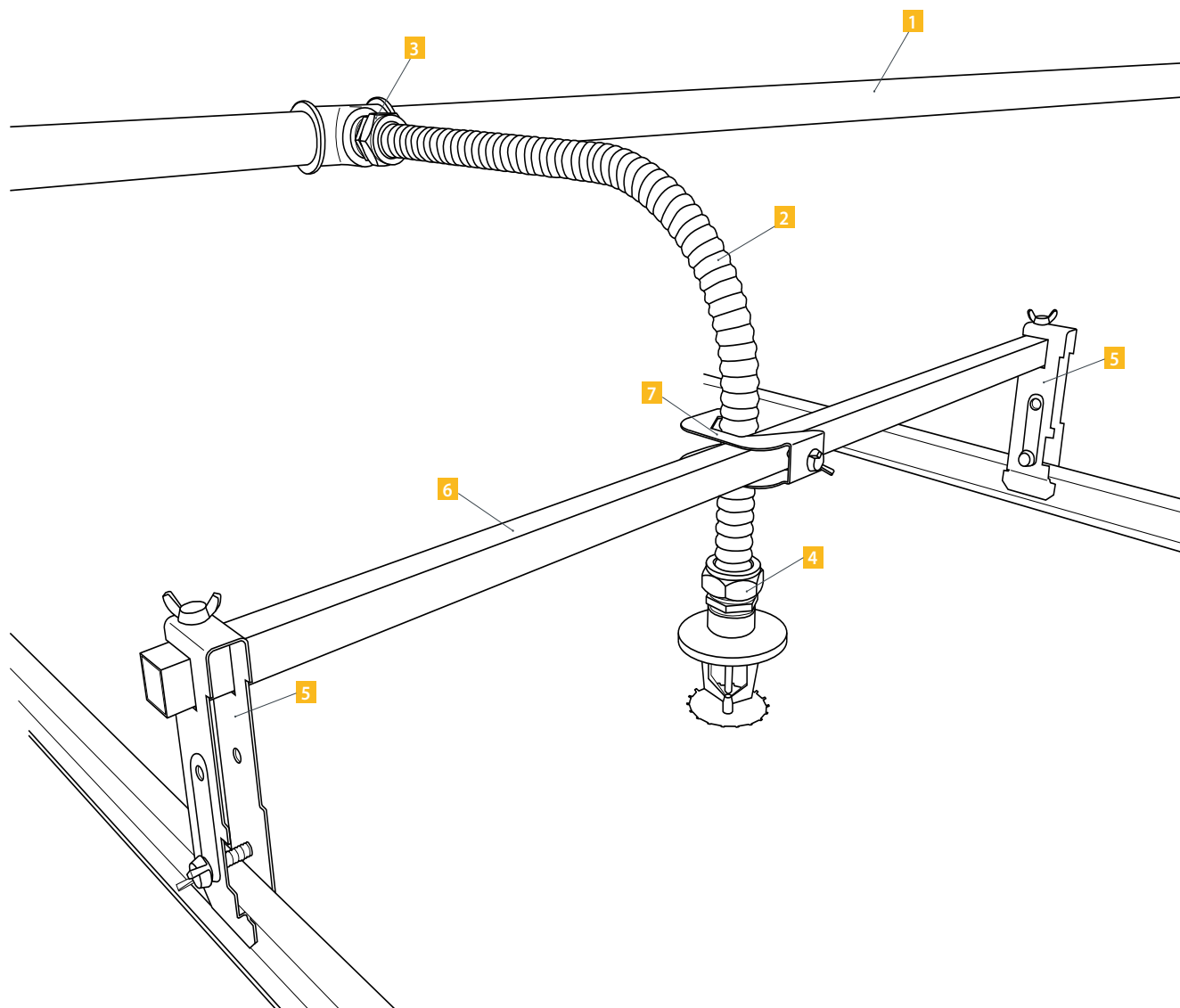
Схема сборки системы креплений Stahlmann для подшивных потолков и потолков типа «Armstrong»
